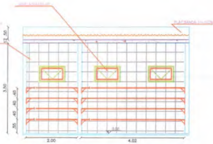
05 | CORTE E-E Escala 1:20
