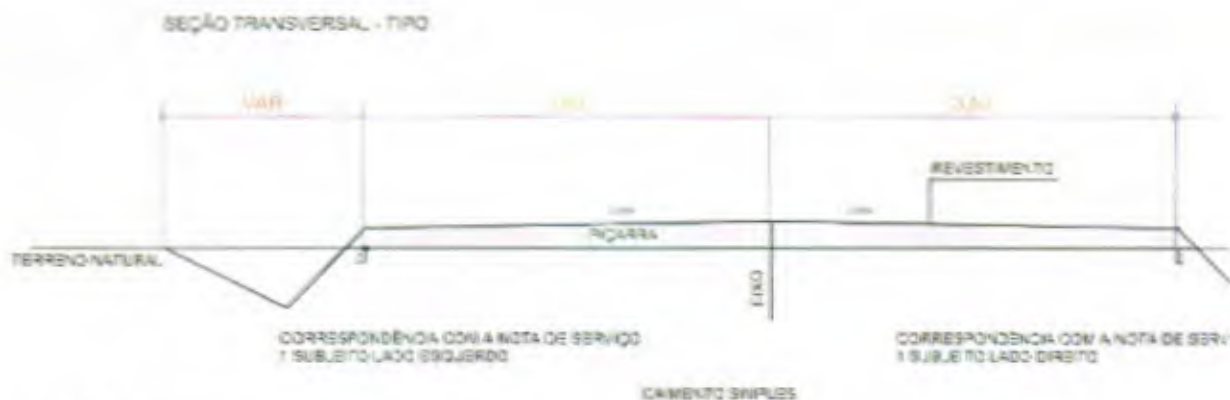
Fig. - Seção tipo da via
