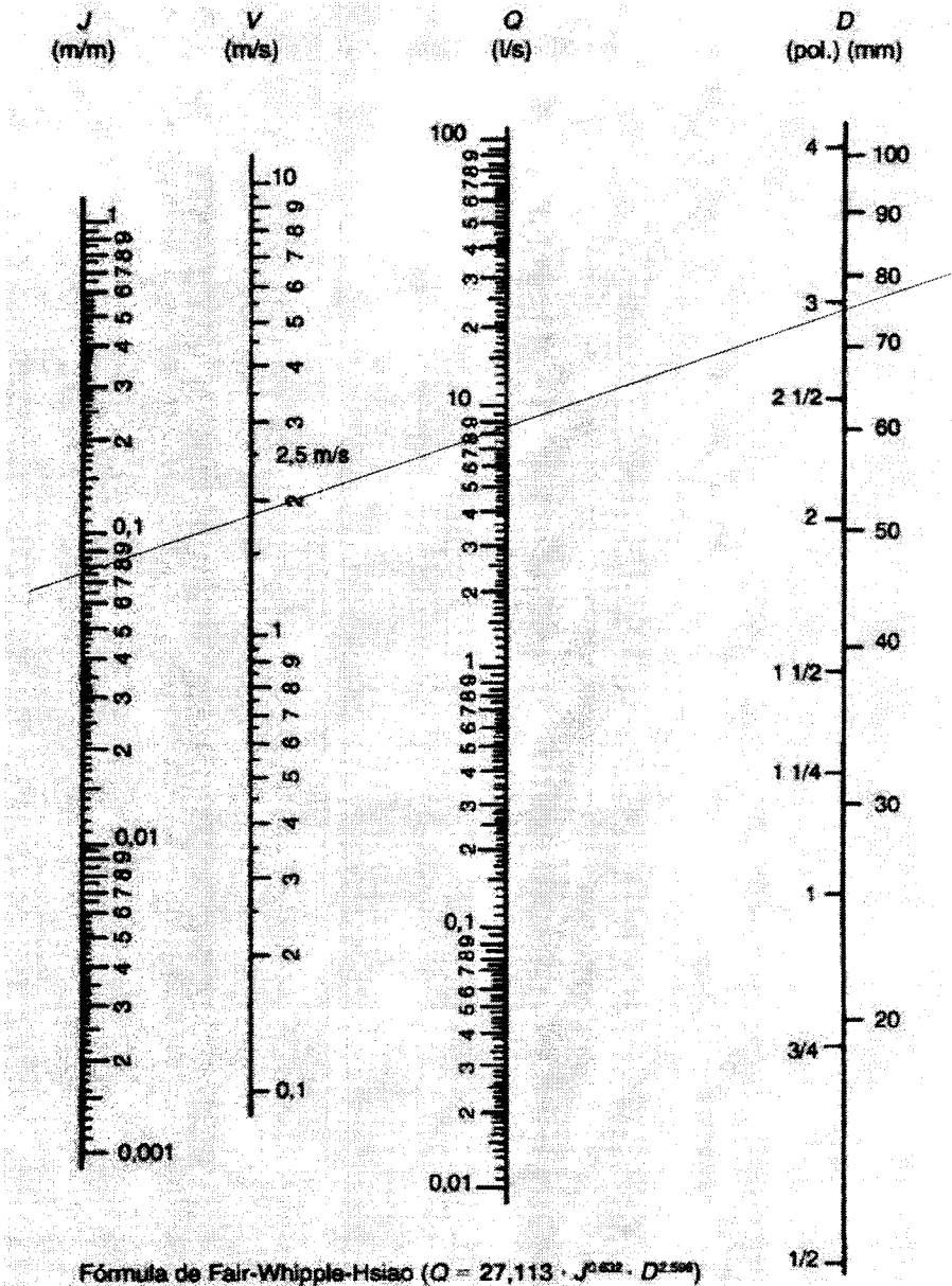
Ábaco para encanamentos de aço galvanizado e ferro fundido. (NBR-5626 – Figura 2.)
